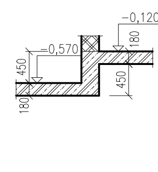
REZ B-B
