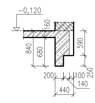
REZ C-C
