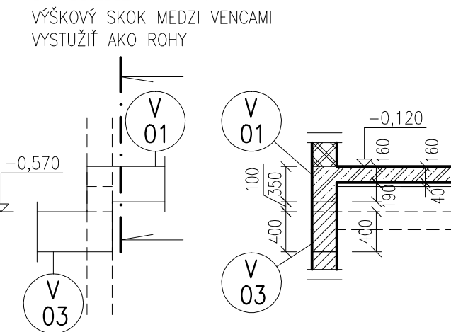
POHLAD G-G
